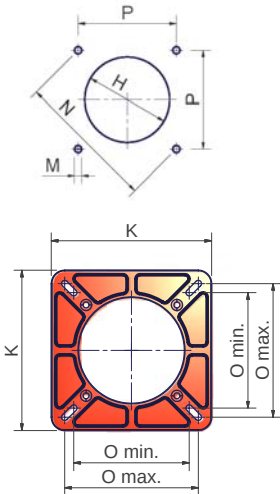
Рис. 3 - Схема для выполнения отверстия в плите котла
