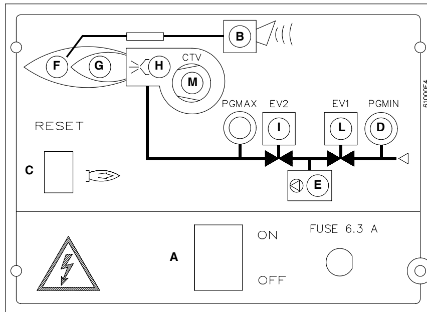
Рис. 28 - Панель управления
